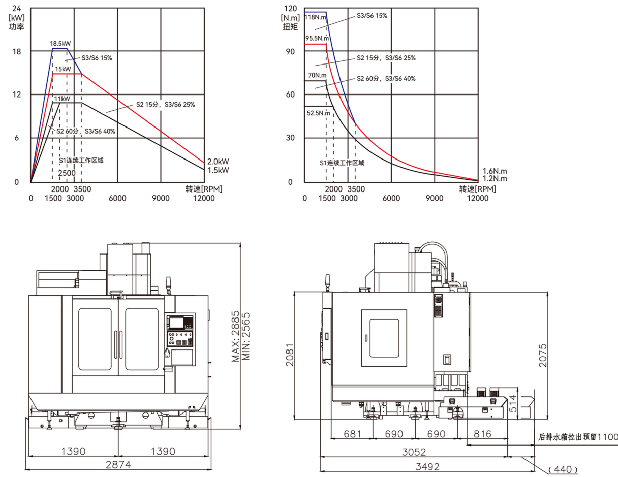
直接/皮带式主轴扭矩
